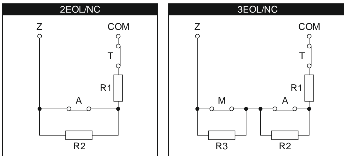
Obr. 11. Číslovanie vyvažovacích rezistorov (pre detektory NO je rovnaká). T – sabotáž. A – alarm. M – masking.
